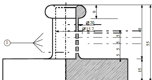
SI.3: Šuplji cilindar; bronca, zatvoren s jedne strane planirati i usjeći dimenzije u mm
