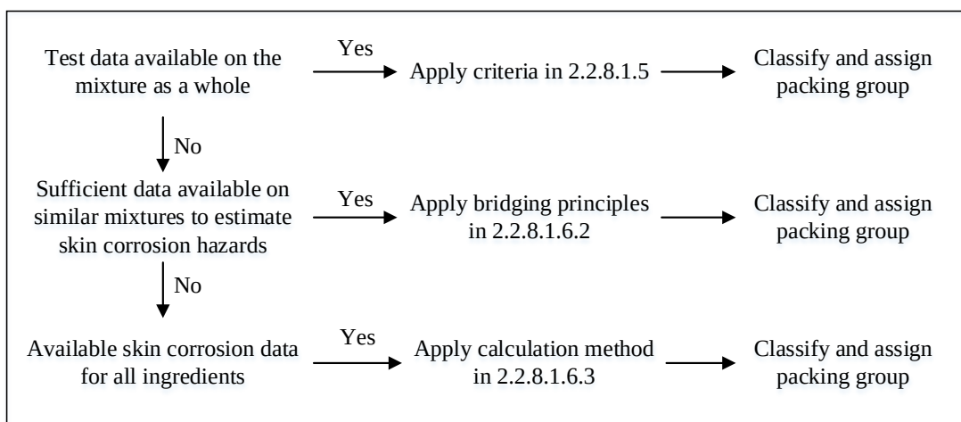
Slika 2.2.8.1.6.1: Koračni pristup klasificiranju i dodjeli ambalažnoj skupini korozivnih smjesa
