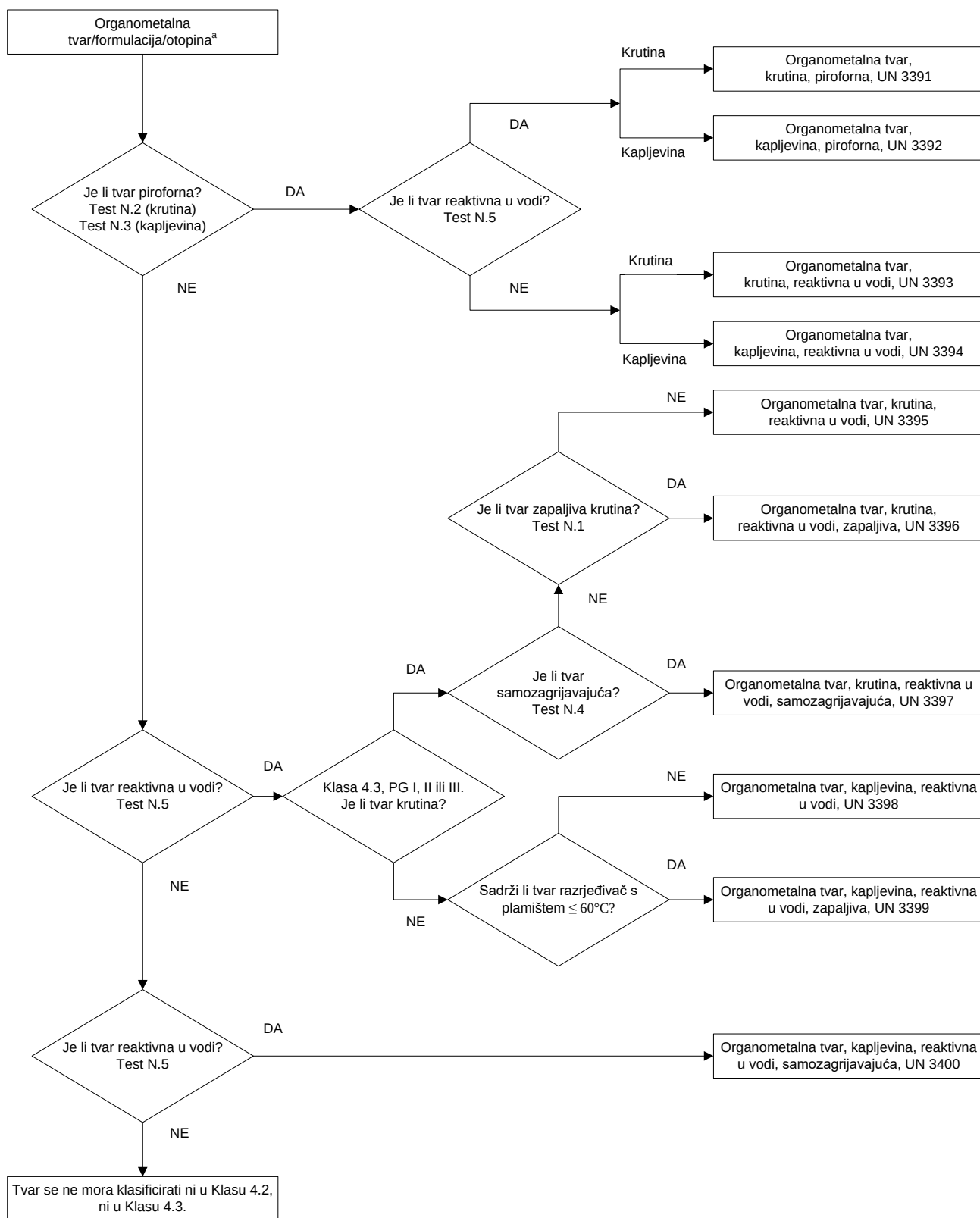
Slika 2.3.5 Shematski prikaz dijagrama toka za klasifikaciju organometalnih tvari u klasama 4.2 i 4.3 b
