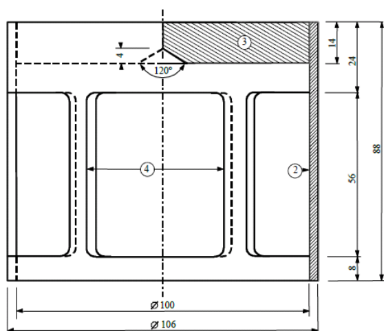
SI.1: Zvonoliki oblik napunjen masom od 2220 g može se objesiti na bronzani klip
