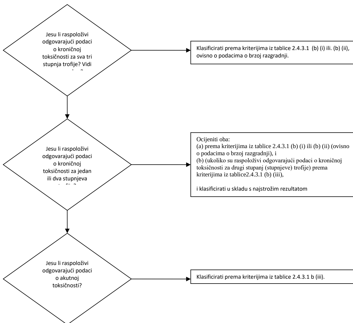
Slika 2.4.3.1: Klasifikacijske kategorije za tvari koje su dugoročno opasne za vodeni okoliš
